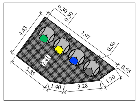
Aikštelės detalizacija
